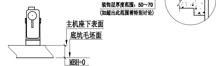
主机座高度示意图
