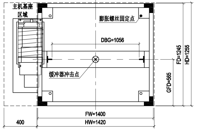
底坑布置图
